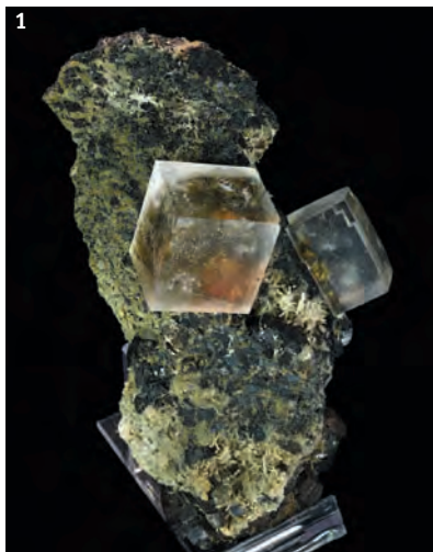
1. Кристаллы флюорита (до 3.5 x 2.5 см) на матрице. 14 x 4 см. Дальнегорск. Образец: В. Пономаренко.
