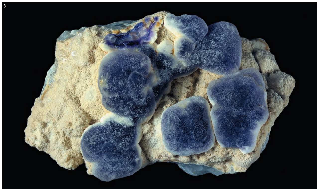
3. Флюорит. 13 x 18 см. Хурайское месторождение, Бурятия. Образец: «Русские минералы».
